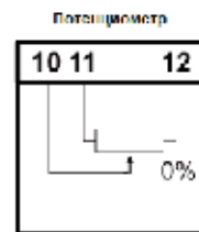
Подключение потенциометра
