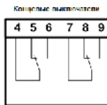
Подключение концевых выключателей
