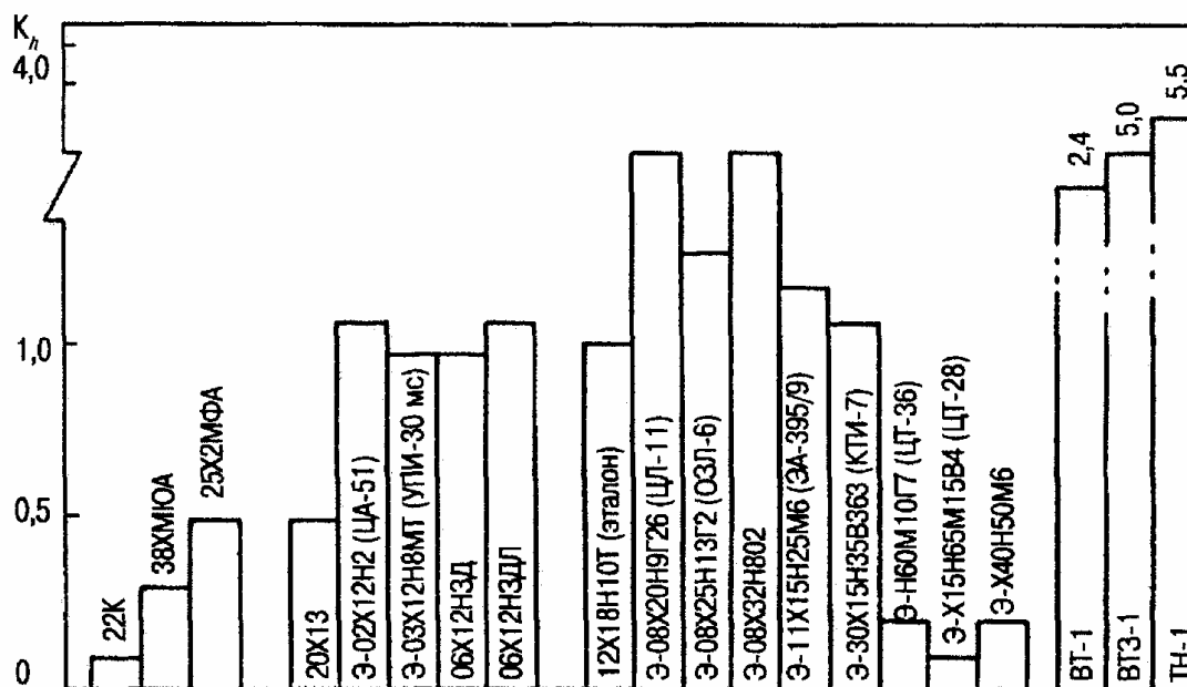
Значения K_h электродуговых наплавочных сталей и титановых сплавов
